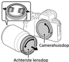
Achterste lensdop
